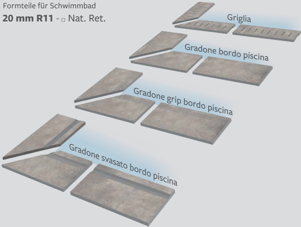
Gradone grip bordo piscina
